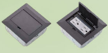
DUFN4000-1 銀灰色薄型地板插座安裝框架 (附自動蓋)
