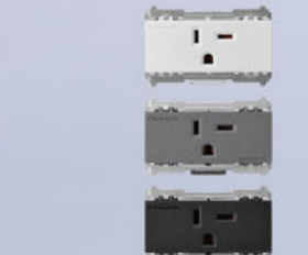
WNF15123MCW(霧白) WNF15123MH(霧灰) WNF15123MB(霧黑) 埋入式瞬間附接地極雙插座 (15A 125V AC)
