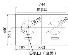
頂視圖
