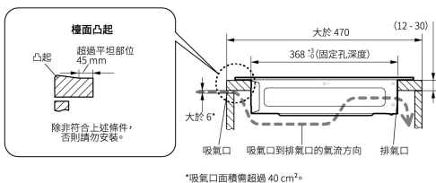
側視圖
