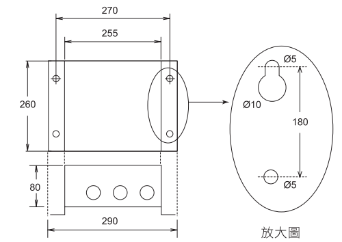
用於各種室外機的串並聯輸入/輸出裝置 (CZ-CAPDC2)
