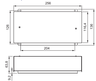
用於各種室內機的串並聯輸入/輸出裝置 (CZ-CAPBC2)
