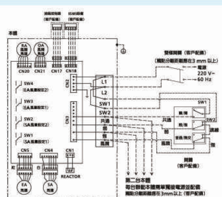
接線配置圖*1
