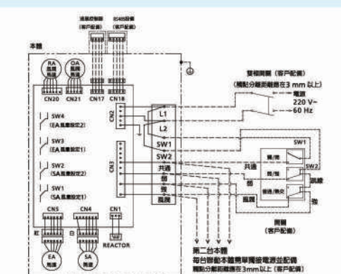
接線配置圖*1
