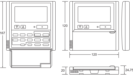
有線遙控器 (CZ-RTC4A)
