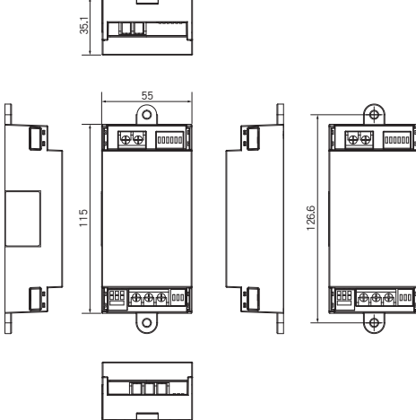
VRF/PAC訊號轉換器 (CZ-T021)
