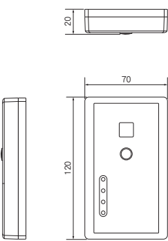
適用於無線遙控器的獨立接收器 (CZ-RWRC3)
