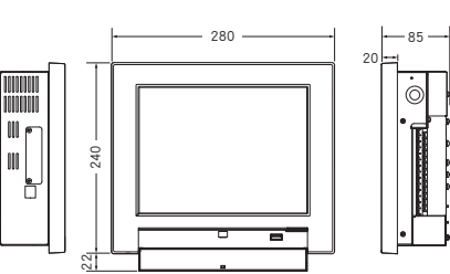
智慧型控制器 (CZ-256ESMC3)
