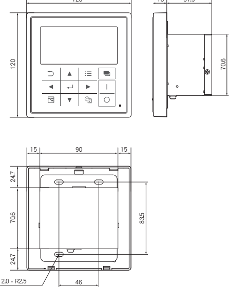
系統控制器 (CZ-64ESMC3)
