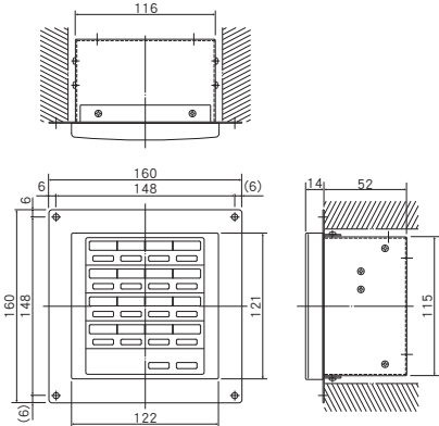
啟閉控制器 (CZ-ANC3)
