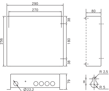
通訊配接器 (CZ-CFUNC2)
