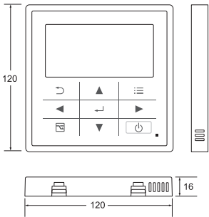
高規格有線遙控器 (CZ-RTC5B)/(CZ-T008)
