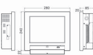
智慧型控制器 (CZ-256ESMC3)
