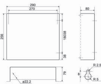
通訊配接器 (CZ-CFUNC2)
