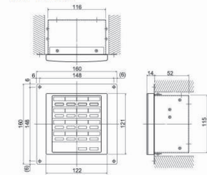
啟閉控制器 (CZ-ANC3)
