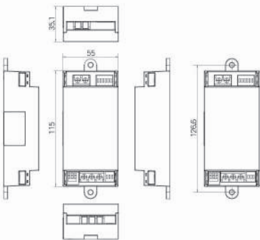
VRF/PAC訊號轉換器 (CZ-T021)
