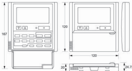
有線遙控器 (CZ-RTC4A)
