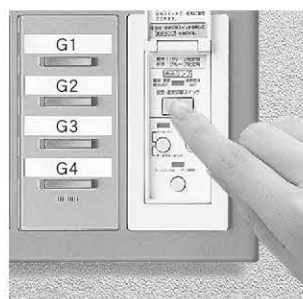
6 群組設定完成時, 按下模式設定按鈕將系統切回正常模式。(紅色LED熄滅)。
