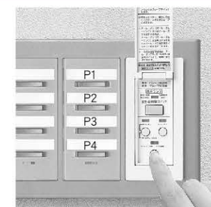
4 在執行初始設定之前, 請先按下重置控制按鈕。(紅色LED亮。) 註: 若您正在確認或執行變更, 切勿執行此步驟4。
