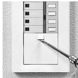
1 鬆開設定單元的蓋板螺絲，將蓋打開。
