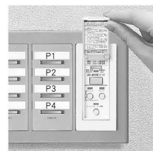
1 打開壁面設定開關 (WRT5850-8) 的蓋板。
