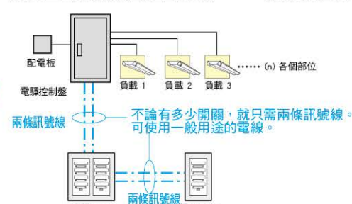
開關僅使用兩條訊號線連接。此兩條訊號線為無極性，因此不易發生施工上的錯誤。
