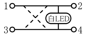
內部迴路圖
