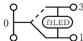
內部迴路圖
