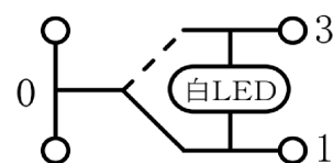
內部迴路圖
