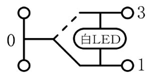
內部迴路圖
