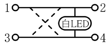
內部迴路圖
