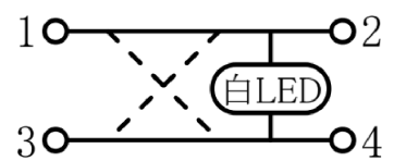
內部迴路圖
