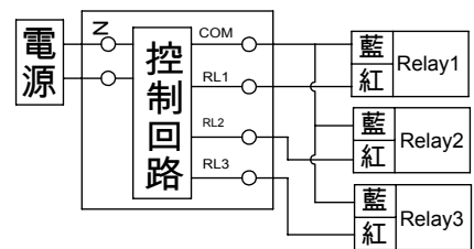
接線圖
