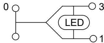
內部回路圖(開關)
