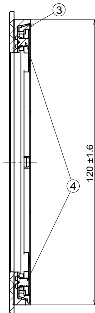
剖面圖 A-A
