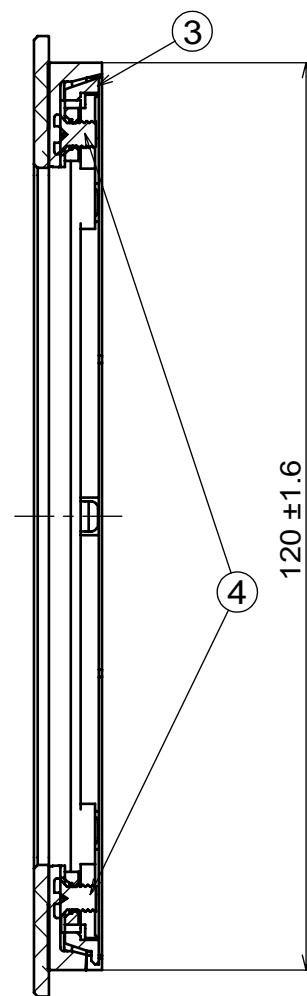
剖面圖 A-A
