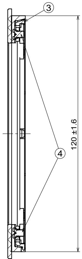
剖面圖 A-A
