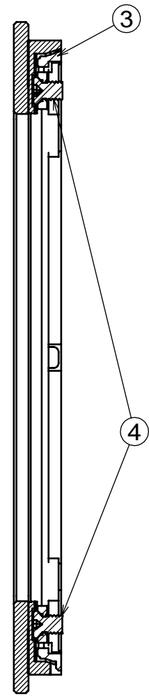
剖面圖 A-A
