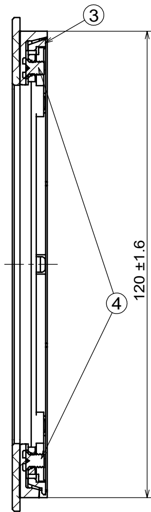
剖面圖 A-A
