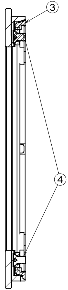
剖面圖 A-A
