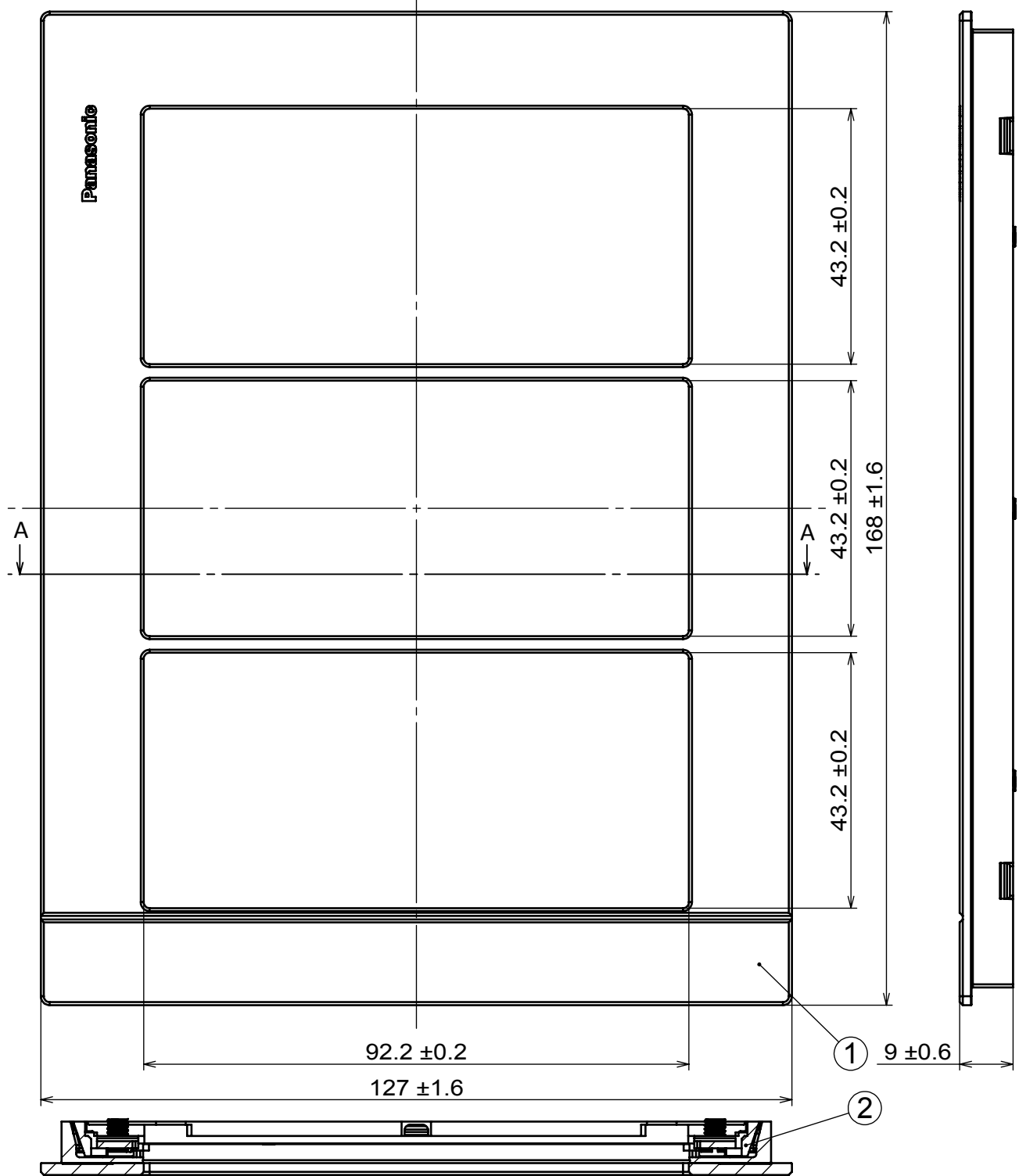
剖面圖 A-A
