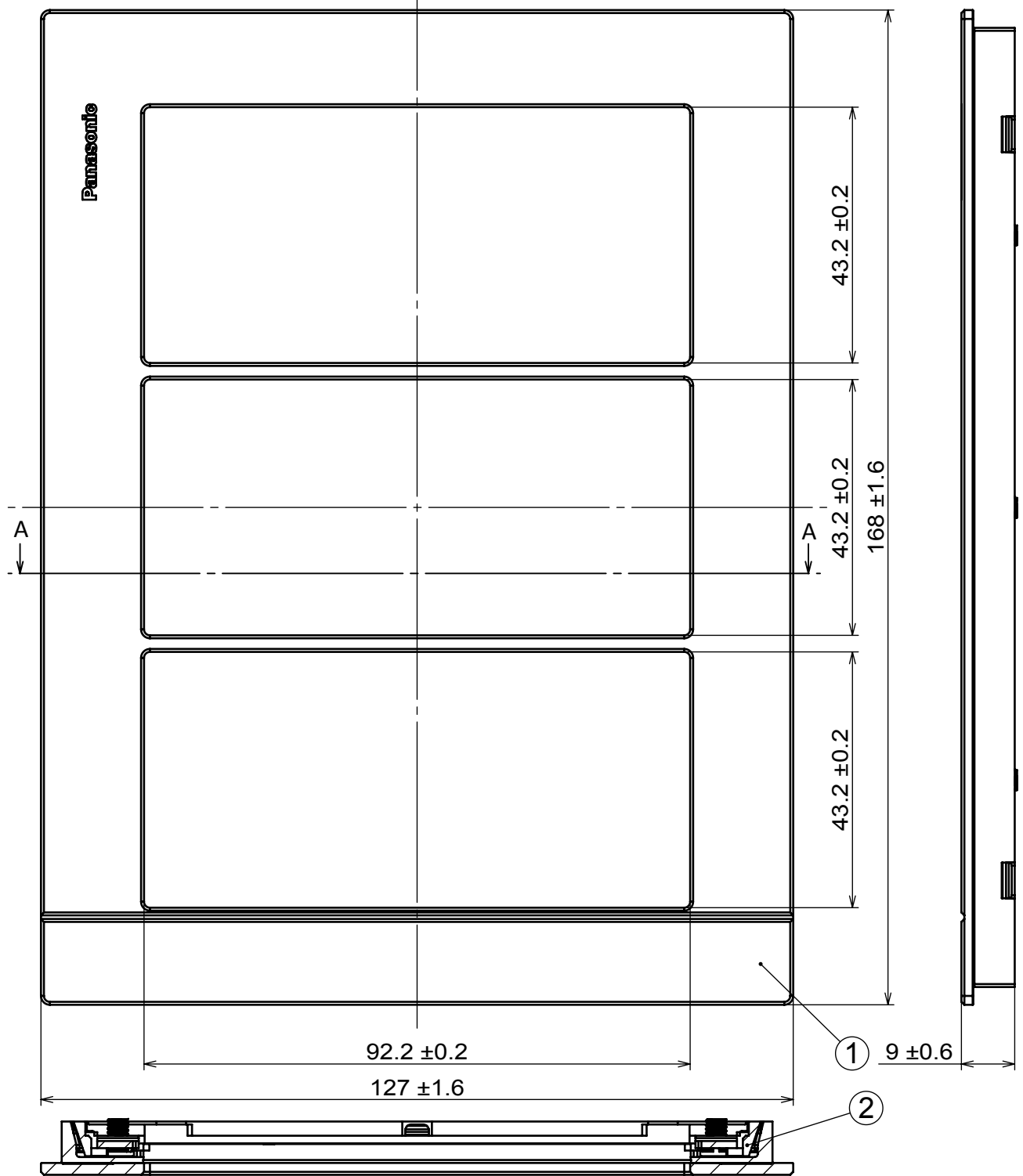
剖面圖 A-A
