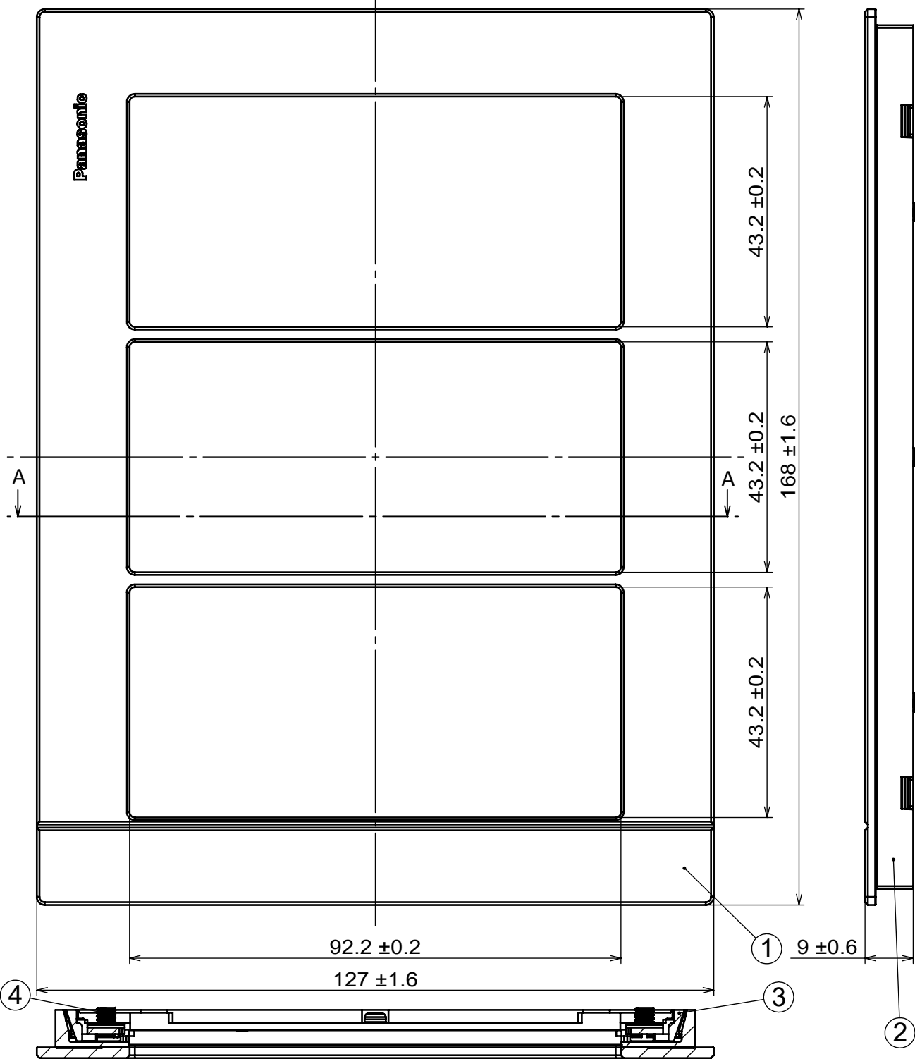
剖面圖 A-A
