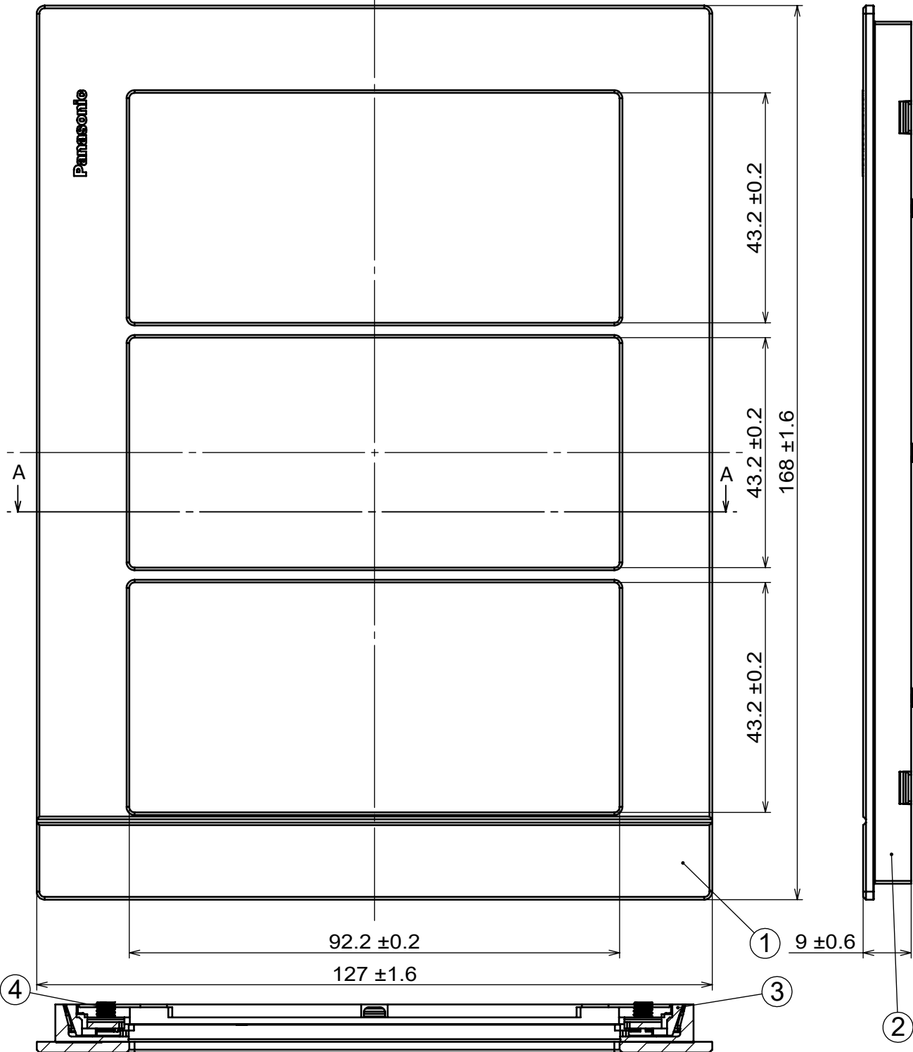
剖面圖 A-A
