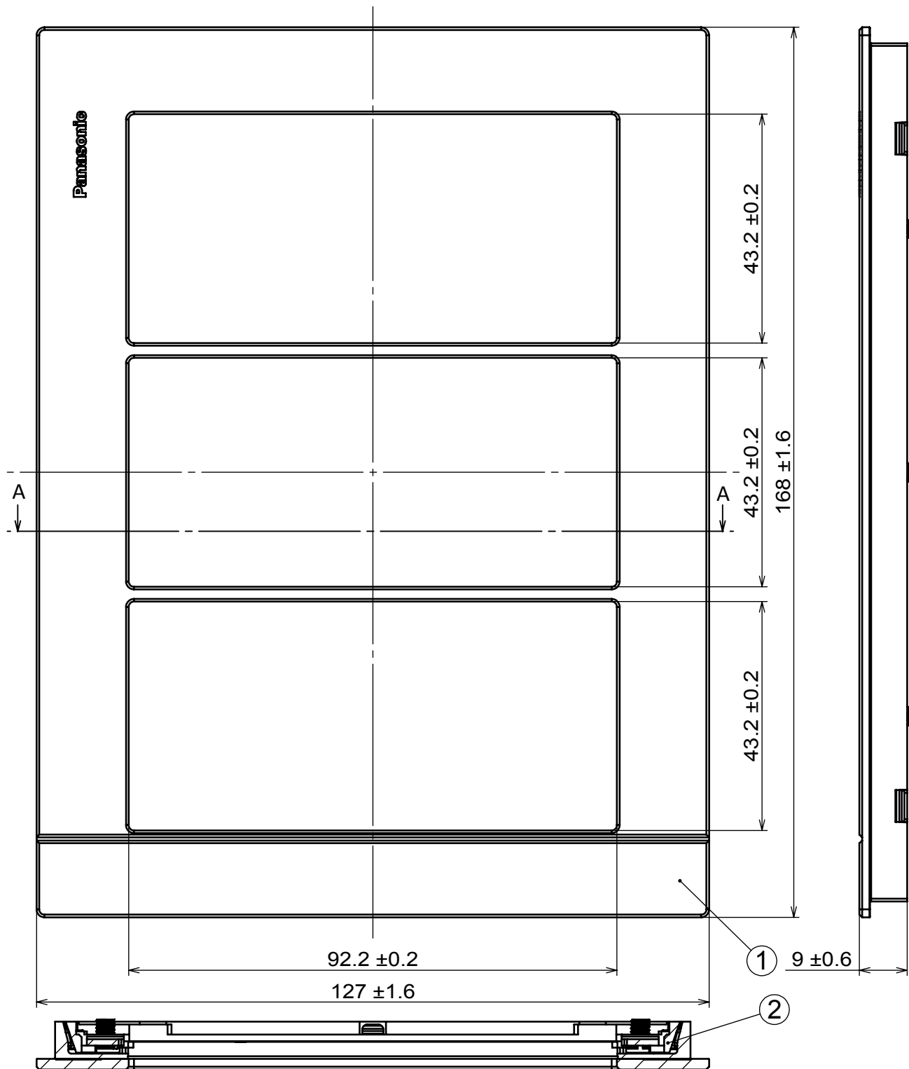
剖面圖 A-A
