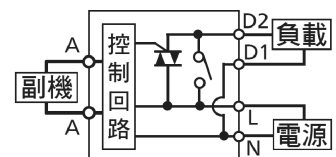
▼內部回路圖
