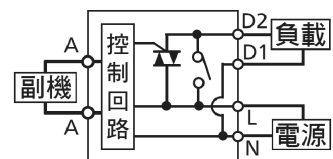
▼內部回路圖
