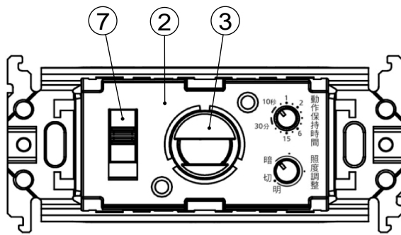
▲外蓋拆除後
