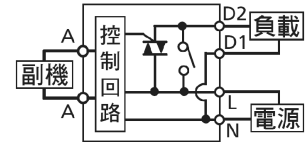
▼內部回路圖
