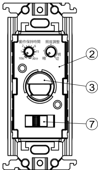
▲外蓋拆除後
