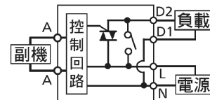
▼內部回路圖
