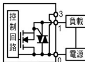
▼內部接線圖
