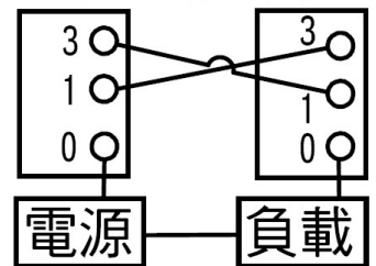
▼2台熱感接續方式
