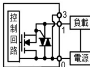
▼內部接線圖
