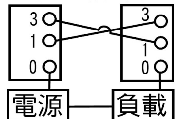
▼2台熱感接續方式
