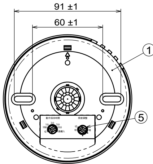
面板拆除後
