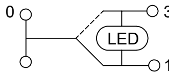
內部迴路圖(開關)
