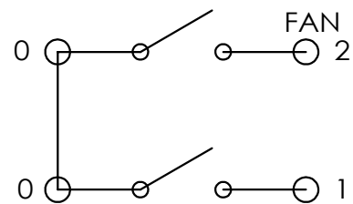
內部迴路圖
