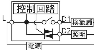
▼ 內部回路圖
