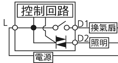
▼內部回路圖
