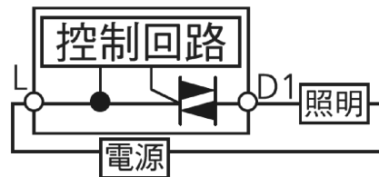
▼ 內部回路圖
