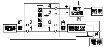
內部回路圖
