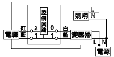
內部回路圖
