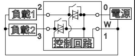
內部回路圖
