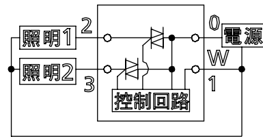
內部回路圖
