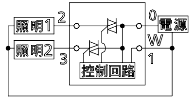
內部回路圖
