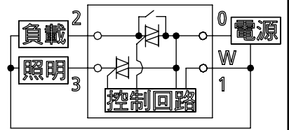
內部回路圖
