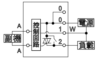
內部回路圖
