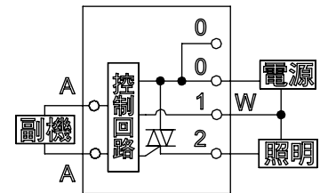
內部回路圖
