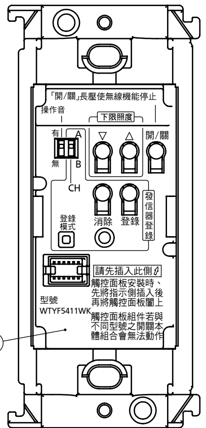
取下觸控面板組件
