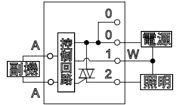
內部回路圖
