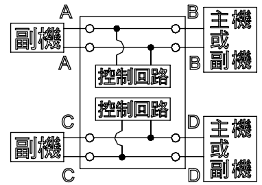
內部回路圖
